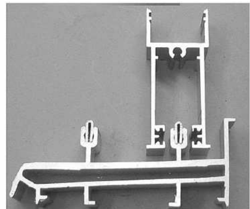
Coupe traverse
